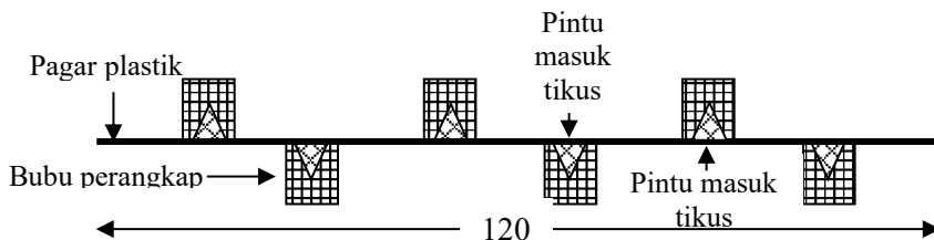
Gambar 18. Skema posisi pemasangan bubu perangkap
